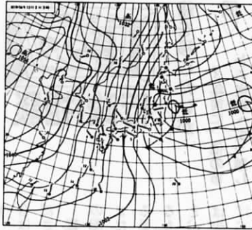
西高東低型の天気図
